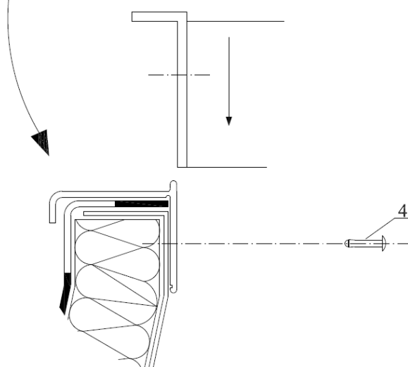
Rys. 8. Montaż napędu klapki dymowej
