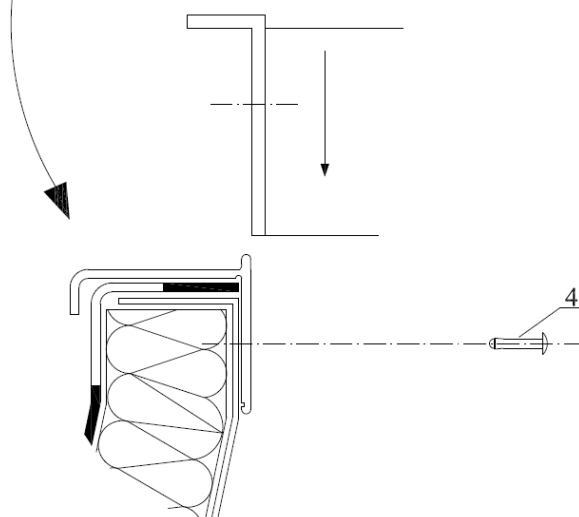
Rys. 8. Montaż napędu kłapy dymowej
