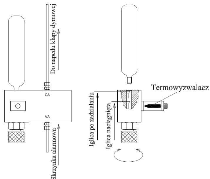
Rys.11. Sposób podłączenia wyzwalacza termicznego i zamykania klap dymowych AWAK
