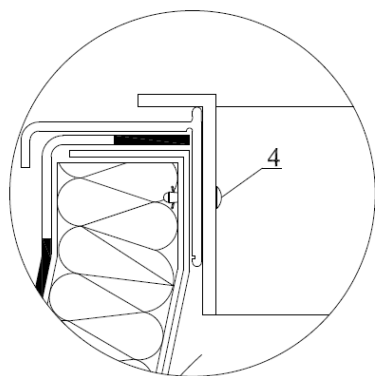
Szczegół A
