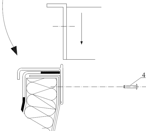
Rys. 7. Montaż napędu klapki dymowej
