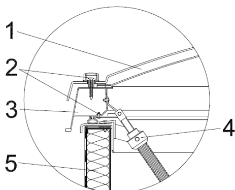
Szczegół A
