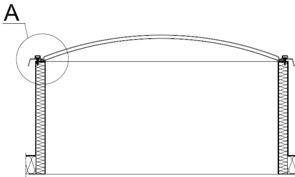
Rys. 1. Światlik stały AWAK - podstawa z blachy stalowej
