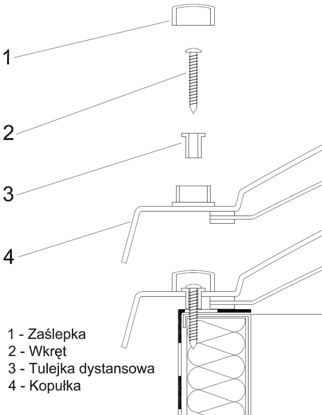
Rys. 11.1. Mocowanie kopułki – świetlik stały
