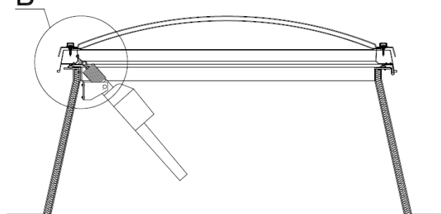
B Podstawa skośna
